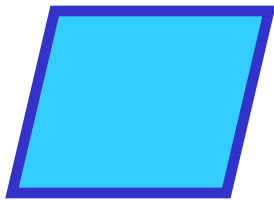
Rhombus
